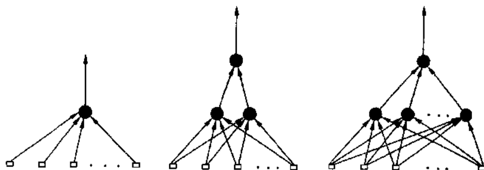
图 4.3 由隐单元数目确定的一种结构
