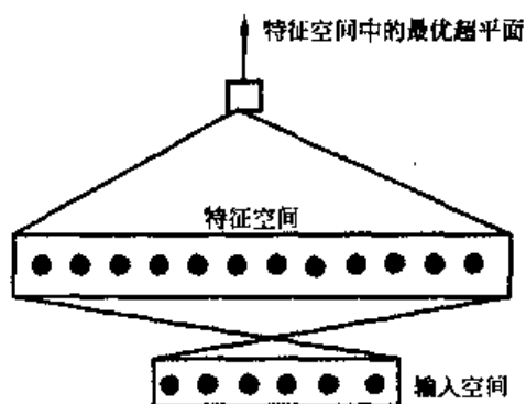
图 5.3 支持向量机把输入空间映射到一个高维特征空间, 然后在这个特征空间中构造最优超平面
