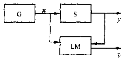
图 1.1 根据样本学习的一个模型。在学习过程中,学习机器 LM 观察数据对 (\mathbf{x}, y) (训练集)。在训练之后,学习机器必须对任意输入 \mathbf{x} 给出输出 \hat{y} 。学习的目标是能够给出输出 \hat{y} , 使之接近训练器的响应 y
