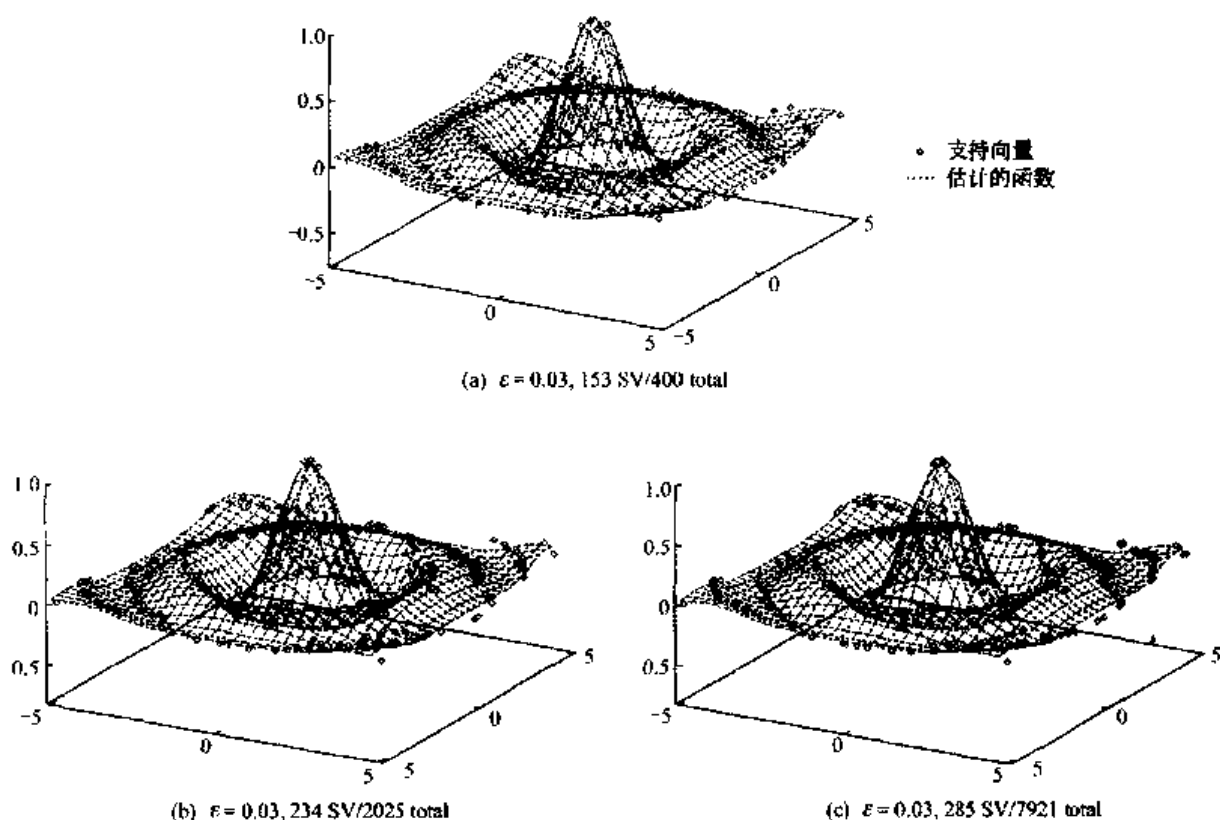
图 6.6 在同一精度( \epsilon=0.03 )下对二次 sinc 函数逼近的结果 (图中“153SV/400 total”表示总共 400 个样本中有 153 个支持向量,余类推)
