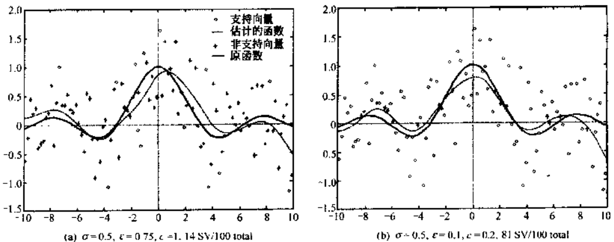
图 6.9 回归函数和对它的逼近
