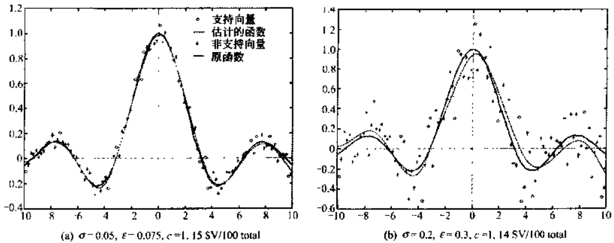
图 6.8 回归函数和对它的逼近
