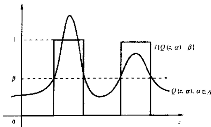
图 3.1 函数 Q(z, \alpha) 的 \beta 水平指示器指示出了 z 为哪些值时, 函数 Q(z, \alpha) 超出了 \beta , 为哪些值时则没有超出。函数 Q(z, \alpha) 可以用其所有指示器的集合来描述
