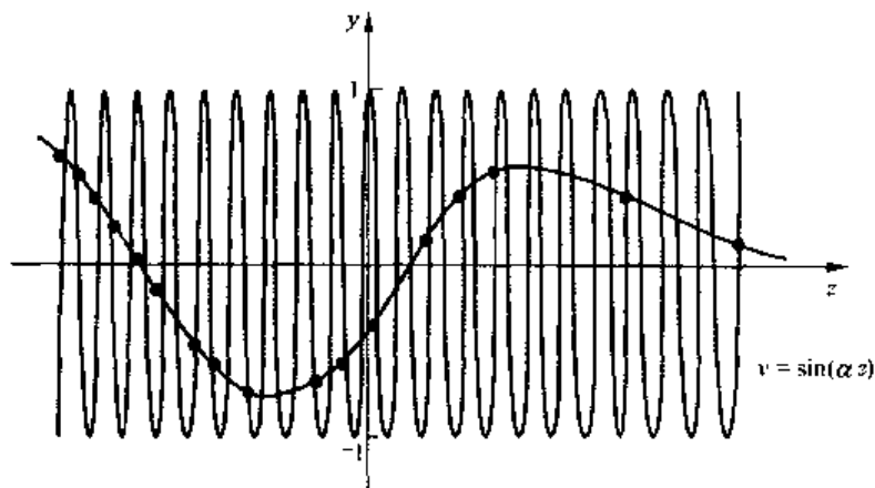
图 3.4 用一个高频函数 \sin(\alpha x) , 我们可以在任何 l 个适当选择的点上很好地逼近任何函数 -1 \leq f(x) \leq 1 的取值
