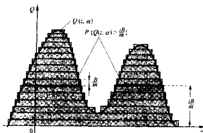
图 2.10 (2-18)式定义的 Lebesgue 积分是一个乘积之和的极限,其中
