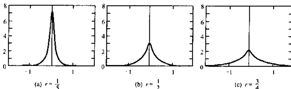
图 6.4 不同 r 值的弱方式正则化的核
