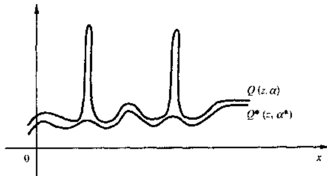
图 2.5 对任意函数 Q(z, \alpha), \alpha \in \Lambda , 考虑一个函数 Q^*(z, \alpha^*), \alpha^* \in \Lambda^* , 它不超出 Q(z, \alpha) 而且与之非常接近
