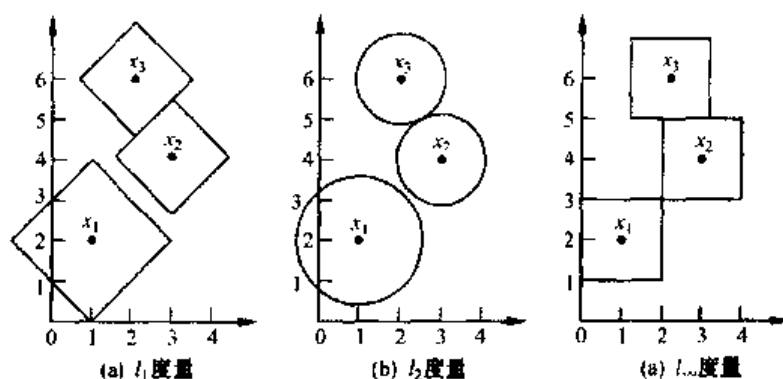
图 8.1 不同度量下点的邻域
