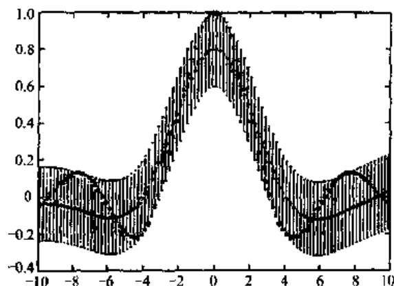
图 6.7 函数逼近的 \epsilon 管道模型 ( \epsilon=0.2 )
