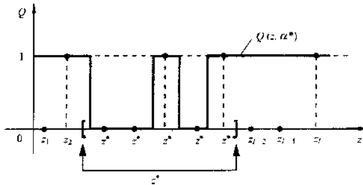
图 2.7 一个采用函数集 Q(z, \alpha), \alpha \in \Lambda 的学习机器, 如果存在一个非零测度的区域 Z^* \in Z , 使得对样本产生器给出的几乎所有样本 z_1, \dots, z_l 及对这些 z 的所有可能的标号 \delta_1, \dots, \delta_l , 机器中总包含一个函数 Q(z, \alpha^*) 对区域 Z^* 中的所有 z , 满足 \delta_i = Q(z_i, \alpha^*), i = 1, \dots, l , 那么这个学习机器是部分不可证伪的。(原著中误写为 \delta_i = Q(z_i, \alpha) ——译者)
