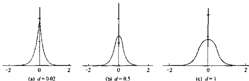
图 8.2 从拉普拉斯函数得到的单邻域核( \Delta=0.25 )
