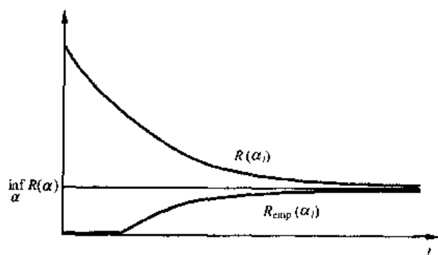
图 2.1 如果期望风险 R(\alpha_l) 和经验风险 R_{\text{emp}}(\alpha_l) 都收敛到最小可能的风险值 \inf_{\alpha \in A} R(\alpha) , 则学习过程是一致的
