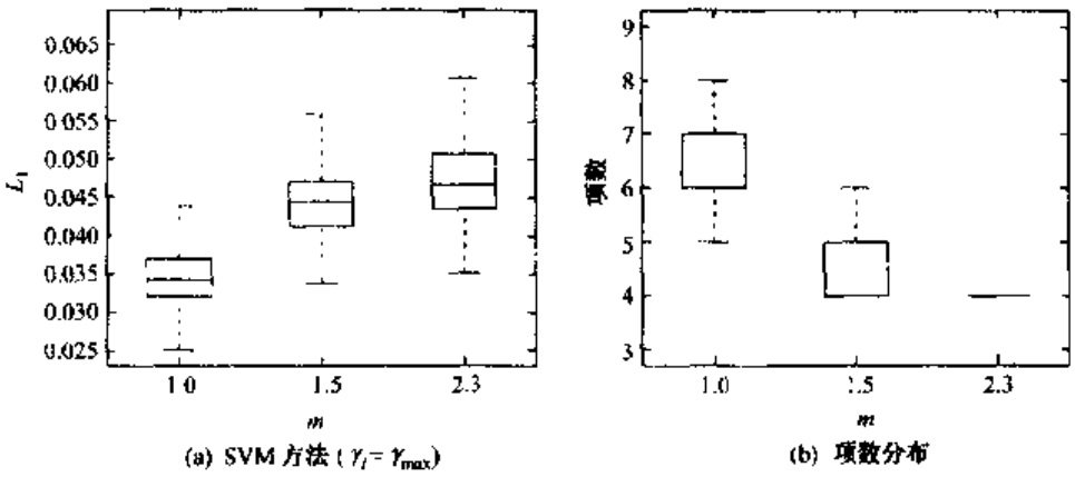
图 7.2 采用 \gamma_i=\gamma_{\max} 的 SVM 方法得到的 L_1 误差及项数分布图 (3 组结果分别是用 \sigma_i=mq/\sqrt{l} 和 m=1.0 , m=1.5 及 m=2.3 得到的)
