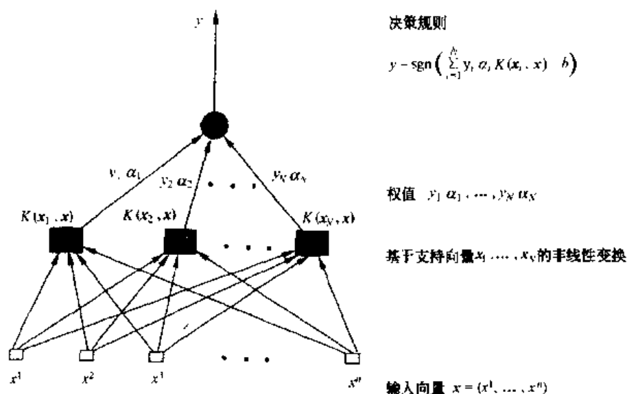
图 5.4 两层的 SV 机是在高维特征空间 Z 中 最优超平面的一个紧凑的实现①
