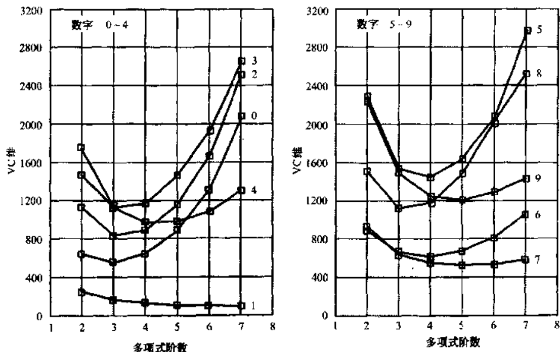
图 5.8 对各个两类数字识别问题(区分某指定数字与其他),(对在相应的特征空间中定义在正规超平面集合上的)结构中最佳元素的 VC 维估计,与多项式阶数之间的关系
