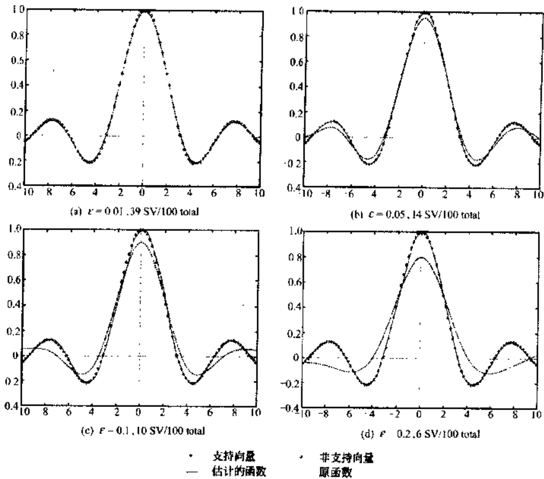
图 6.5 不同精度要求的逼近需要不同数目的支持向量 (图中“39SV/100 total”表示总共 100 个样本中有 39 个支持向量,余类推)
