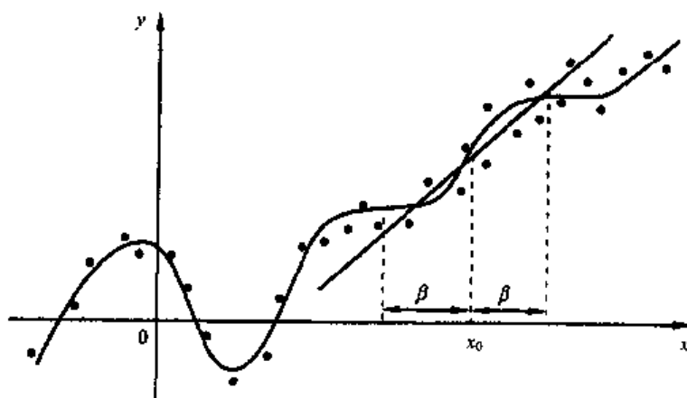
图 4.5 用线性函数,我们可以在所关心的任意点的近邻内估计未知的平滑函数
