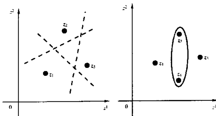
图 3.3 平面中直线的 VC 维等于 3, 因为它们能打散 3 个向量而不能打散 4 个: 例如向量 z_2, z_4 不能被直线与向量 z_1, z_3 分开
