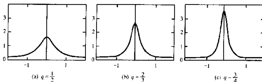
图 6.3 不同 q 值的强方式正则化的核
