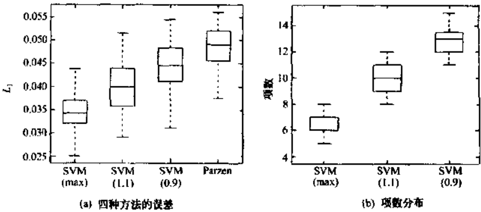
图 7.1 用不同方法得到的 L_1 误差和项数分布图 (4 种方法是 \gamma_i=\gamma_{\max} , \gamma_i=1.1 , \gamma_i=0.9 的 SVM 方法及 Parzen 方法)
