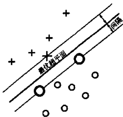
图 5.2 最优分类超平面是以最大间隔将数据分开的超平面
