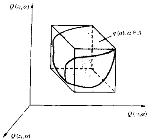
图 2.4 l 维向量集合 q(\alpha), \alpha \in \Lambda 处 在一个 l 维立方体之中
