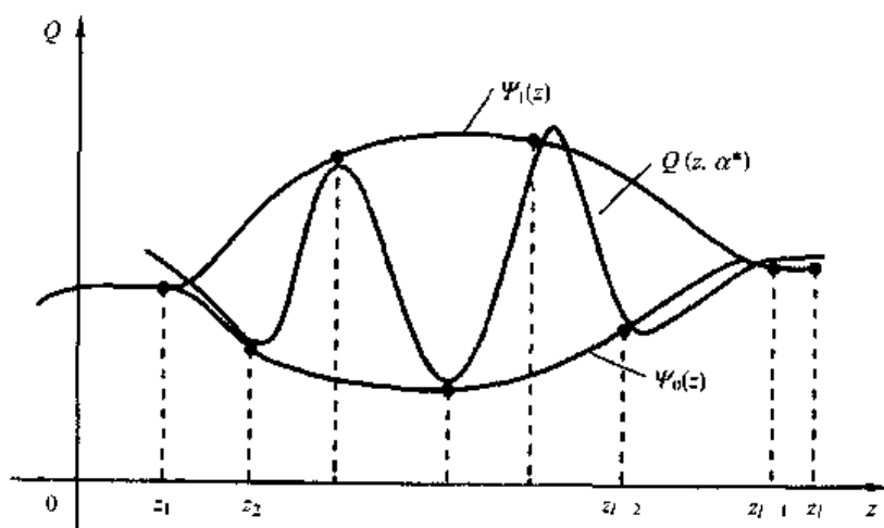
图 2.8 一个函数集为 Q(z, \alpha), \alpha \in \Lambda 的学习机器, 如果对任何 \varepsilon > 0 , 存在两个有实质性差别的函数 \psi_1(z) 和 \psi_0(z) , 使得对样本产生器给出的几乎所有样本 z_1, \dots, z_l , 和用这两个函数及规则 u_i = \psi_{\delta(z_i)}(z_i) 构造的任何取值 u_1, \dots, u_l (其中 \delta(z) \in \{0, 1\} 是任一二值函数), 总有一个函数 Q(z, \alpha^*) 满足不等式 |\psi_{\delta(z_i)}(z_i) - Q(z_i, \alpha^*)| \leq \varepsilon, i = 1, \dots, l , 那么这个学习机器是潜在不可证伪的
