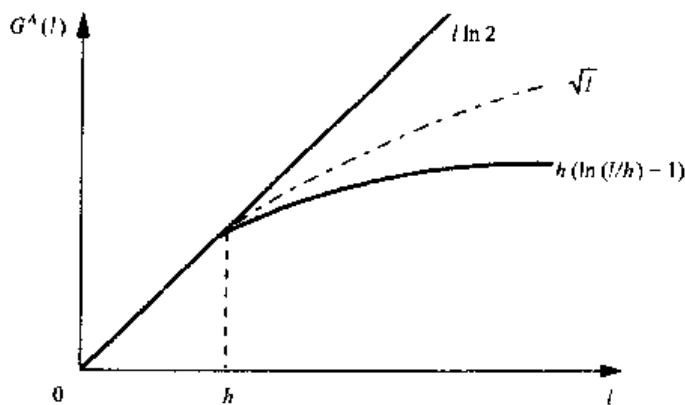
图 3.2 生长函数或者是线性的,或者以一个对数函数为界。 比如,它不可能像图中的点划线那样
