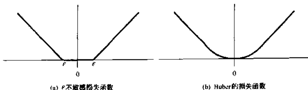
图 6.1 损失函数的比较
