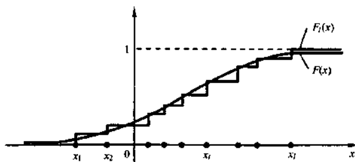
图 1.2 从数据 x_1, \dots, x_l 构造出的经验分布函数 F_l(x) , 它逼近概率分布函数 F(x)
