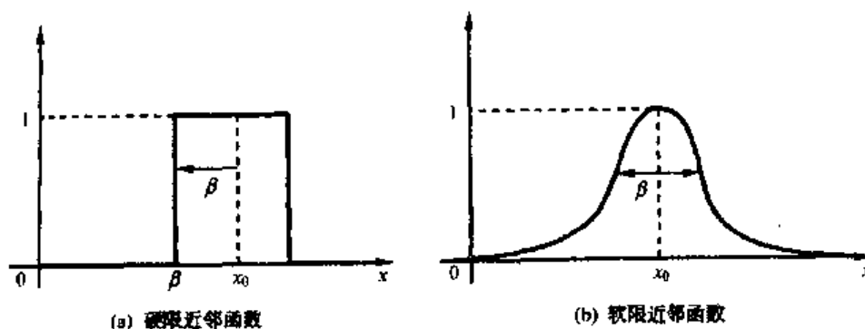
图 4.4 近邻函数的例子
