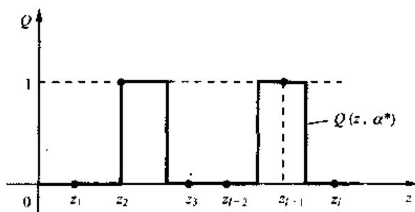
图 2.6 一个采用函数集 Q(z, \alpha), \alpha \in \Lambda 的学习机器,如果对样本产生器给出的几乎所有样本 z_1, \dots, z_l 以及对这些 z 的所有可能的标号 \delta_1, \dots, \delta_l ,机器中总包含一个函数 Q(z, \alpha') 满足 \delta_i = Q(z_i, \alpha') , i = 1, \dots, l , 那么这个学习机器是不可证伪的
