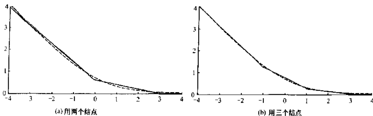
图 5.10 逻辑损失函数(虚线)及其逼近(实线)
