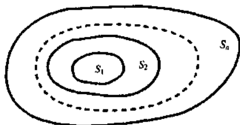
图 4.1 函数集的结构是由嵌套的函数子集确定的
