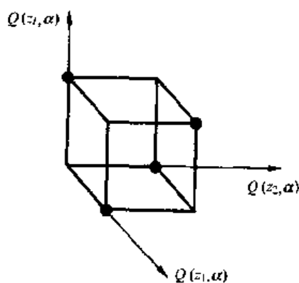
图 2.3 l 维二值向量集合 q(\alpha), \alpha \in \Lambda 是 l 维单位立方体的顶点集合的一个子集
