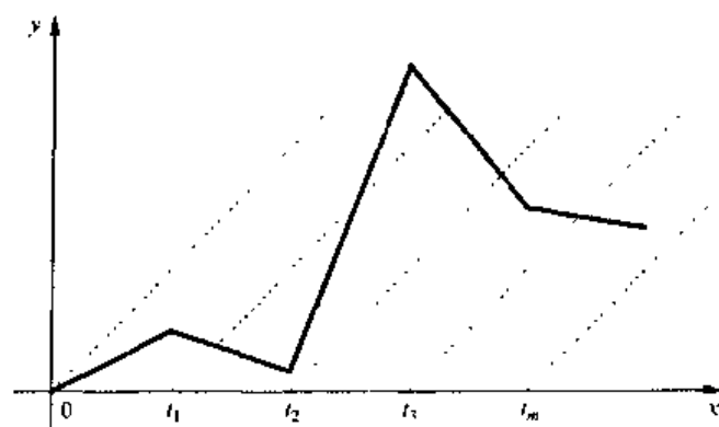
图 6.2 用函数 1, x, (x-t_1)_+, \dots, (x-t_m)_+ 的展开,我们可以构造对一个函数的分段线性逼近。类似地,函数 1, x, \dots, x^d, (x-t_1)_+^d, \dots, (x-t_m)_+^d 的展开提供了分段多项式逼近
