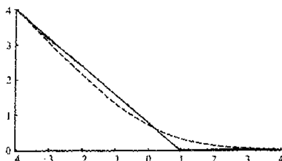
图 5.9 逻辑损失函数(虚线)和用一个结点的线性样条对它的逼近(实线)
