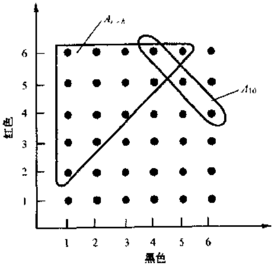
图 2.9 双骰子实验的基本事件空间, 其中标出了事件 A_{10} 和 A_{r>b}
