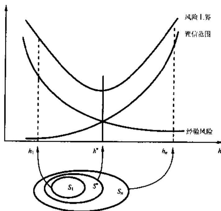
图 4.2 风险的界是经验风险与置信范围之和。随着结构元素序号的增加,经验风险将减小,而置信范围将增加。最小的风险上界是在结构的某个适当的元素上取得的
