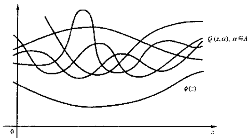
图 2.2 平凡一致性的情况。ERM 方法对函数集 Q(z, \alpha), \alpha \in A 来说不一致，而对函数集 \{\phi(z)\} \cup Q(z, \alpha), \alpha \in A 则一致
